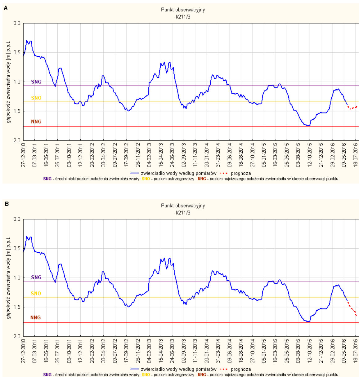
Rys. 13. Prognoza dotycząca stanu wód o zwierciadle swobodnym (gruntowych) na okres 01.07-31.07.2016r. – stacja hydrogeologiczna nr I/211/3 w Brwinowie (woj. mazowieckie). A - prognoza przy założeniu scenariusza A; B - prognoza przy założeniu scenariusza B
