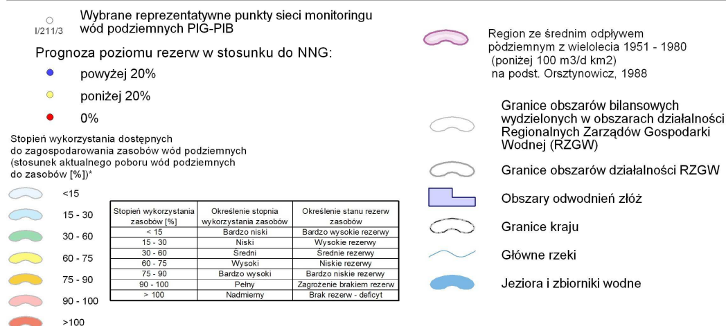
Rys. 33. Prognoza poziomu rezerw wód podziemnych w odniesieniu do najniższego zaobserwowanego w wieloleciu położenia zwierciadła wód (NNG) – lipiec 2016 rok
