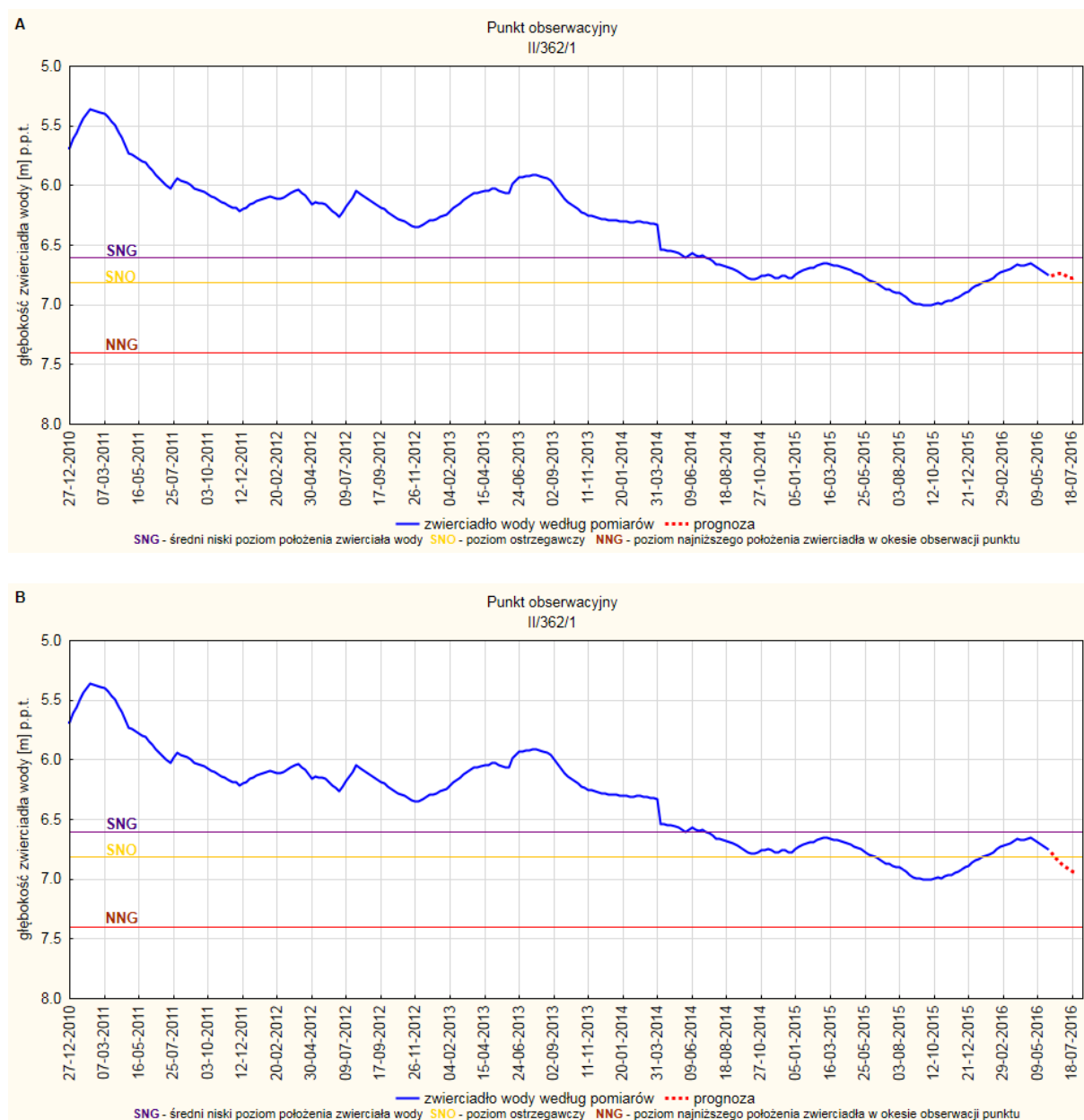
Rys. 4. Prognoza dotycząca stanu wód o zwierciadle swobodnym (gruntowych) na okres 01.07-31.07.2016r. – stacja hydrogeologiczna nr II/362/1 w Słońsku (woj. lubuskie). A - prognoza przy założeniu scenariusza A; B - prognoza przy założeniu scenariusza B
