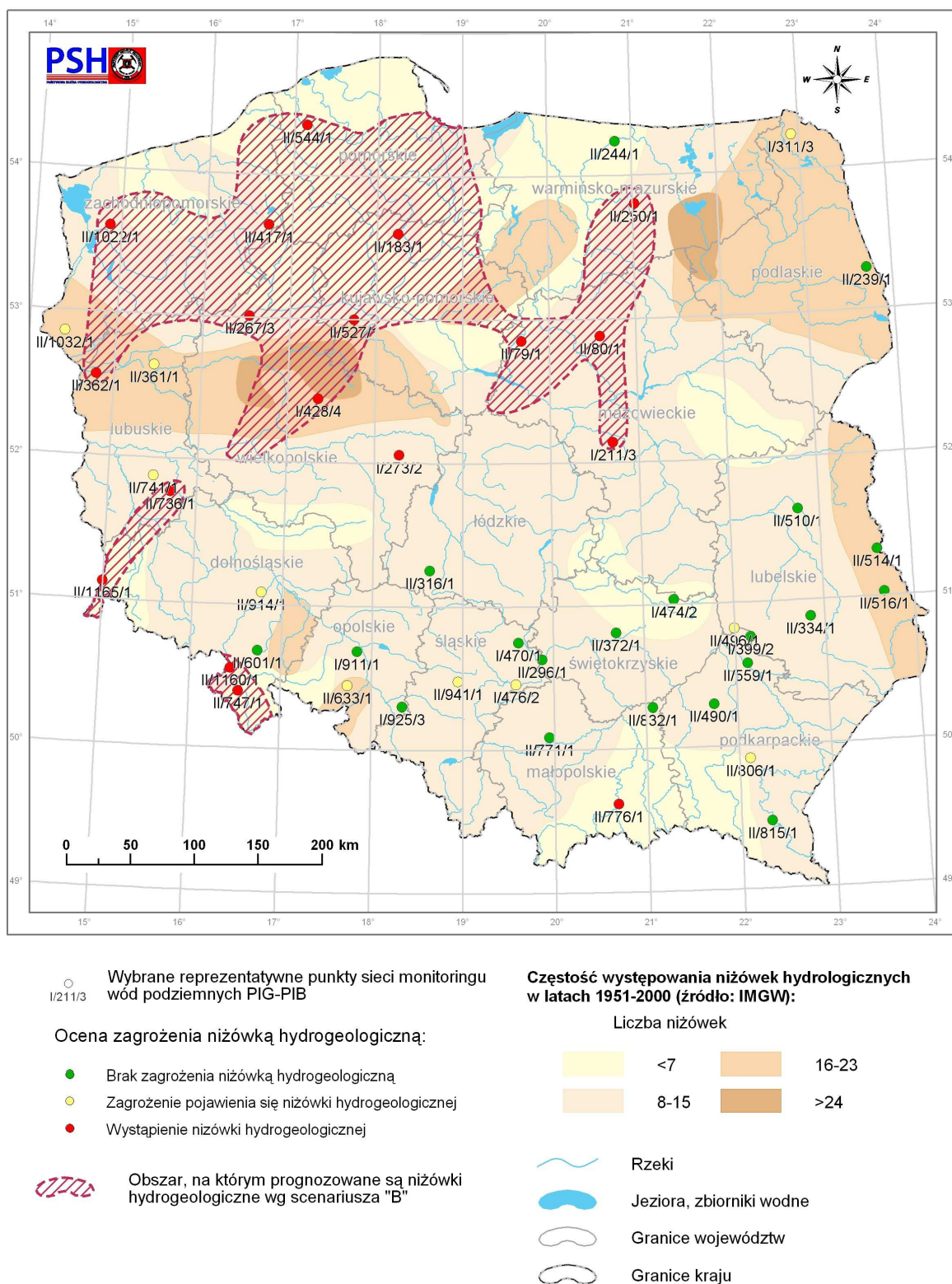
Rys. 34. Prognoza zagrożenia wystąpienia niżówki hydrogeologicznej dla wód podziemnych – lipiec 2016 rok
