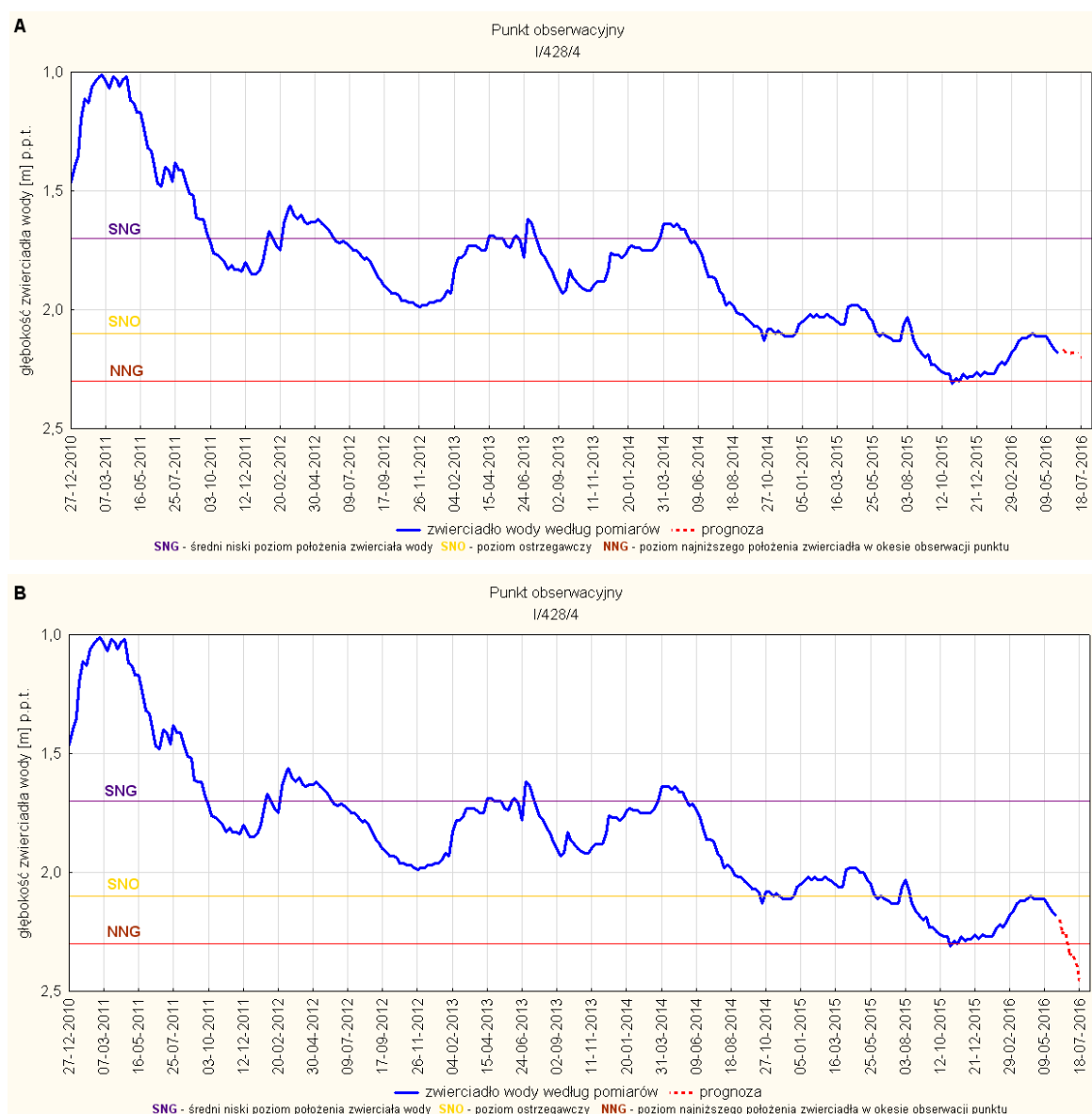
Rys. 10. Prognoza dotycząca stanu wód o zwierciadle swobodnym (gruntowych) na okres 01.07-31.07.2016r. – stacja hydrogeologiczna nr I/428/4 w miejscowości Czachurki (woj. wielkopolskie). A - prognoza przy założeniu scenariusza A; B - prognoza przy założeniu scenariusza B
