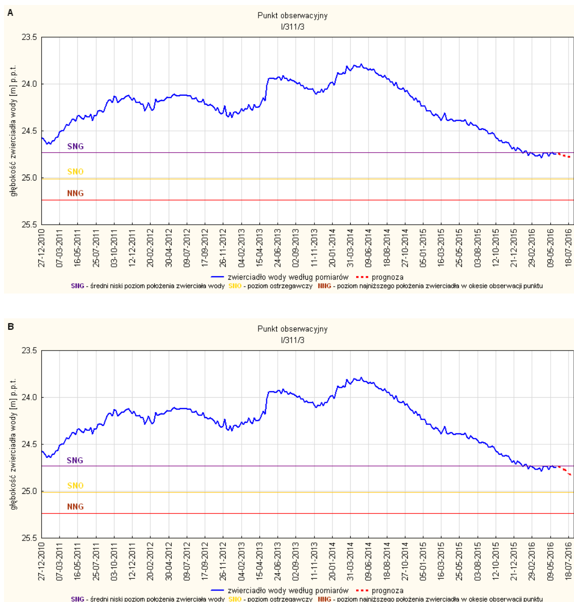
Rys. 7. Prognoza dotycząca stanu wód o zwierciadle swobodnym (gruntowych na okres 01.07-31.07.2016r. - stacja hydrogeologiczna nr I/311/3 w Sidorówce (woj. podlaskie). A - prognoza przy założeniu scenariusza A; B - prognoza przy założeniu scenariusza B
