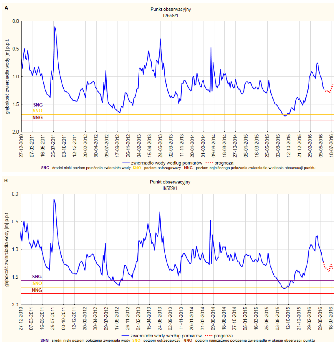
Rys. 19. Prognoza dotycząca stanu wód o zwierciadle swobodnym (gruntowych) na okres 01.07-31.07.2016r. – stacja hydrogeologiczna nr II/559/1 w miejscowości Pysznica (woj. podkarpackie). A - prognoza przy założeniu scenariusza A; B - prognoza przy założeniu scenariusza B,
