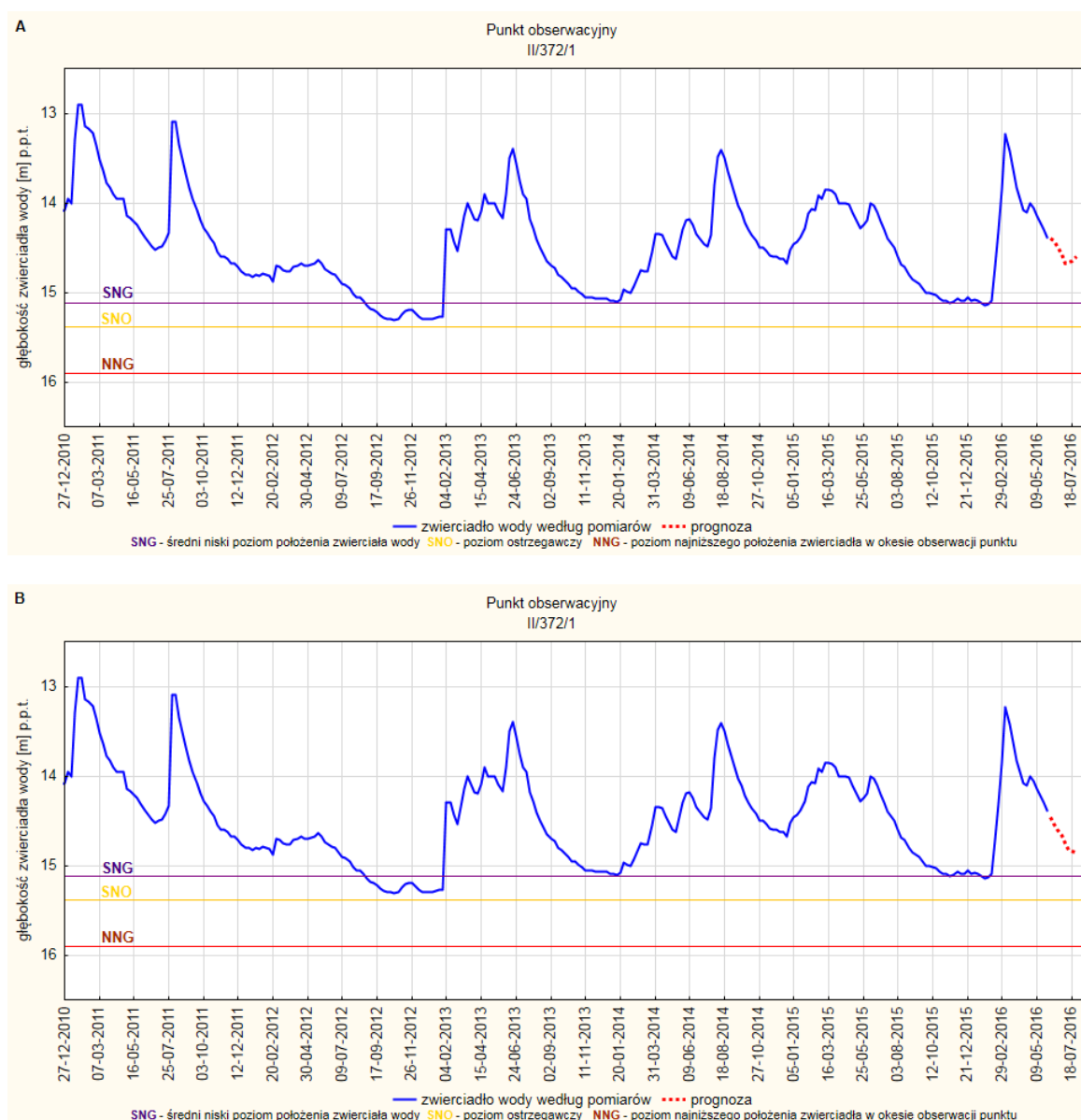
Rys. 8. Prognoza dotycząca stanu wód o zwierciadle swobodnym (gruntowych) na okres 01.07-31.07.2016r. – stacja hydrogeologiczna nr II/372/1 w miejscowości Suków (woj. świętokrzyskie). A - prognoza przy założeniu scenariusza A; B - prognoza przy założeniu scenariusza B
