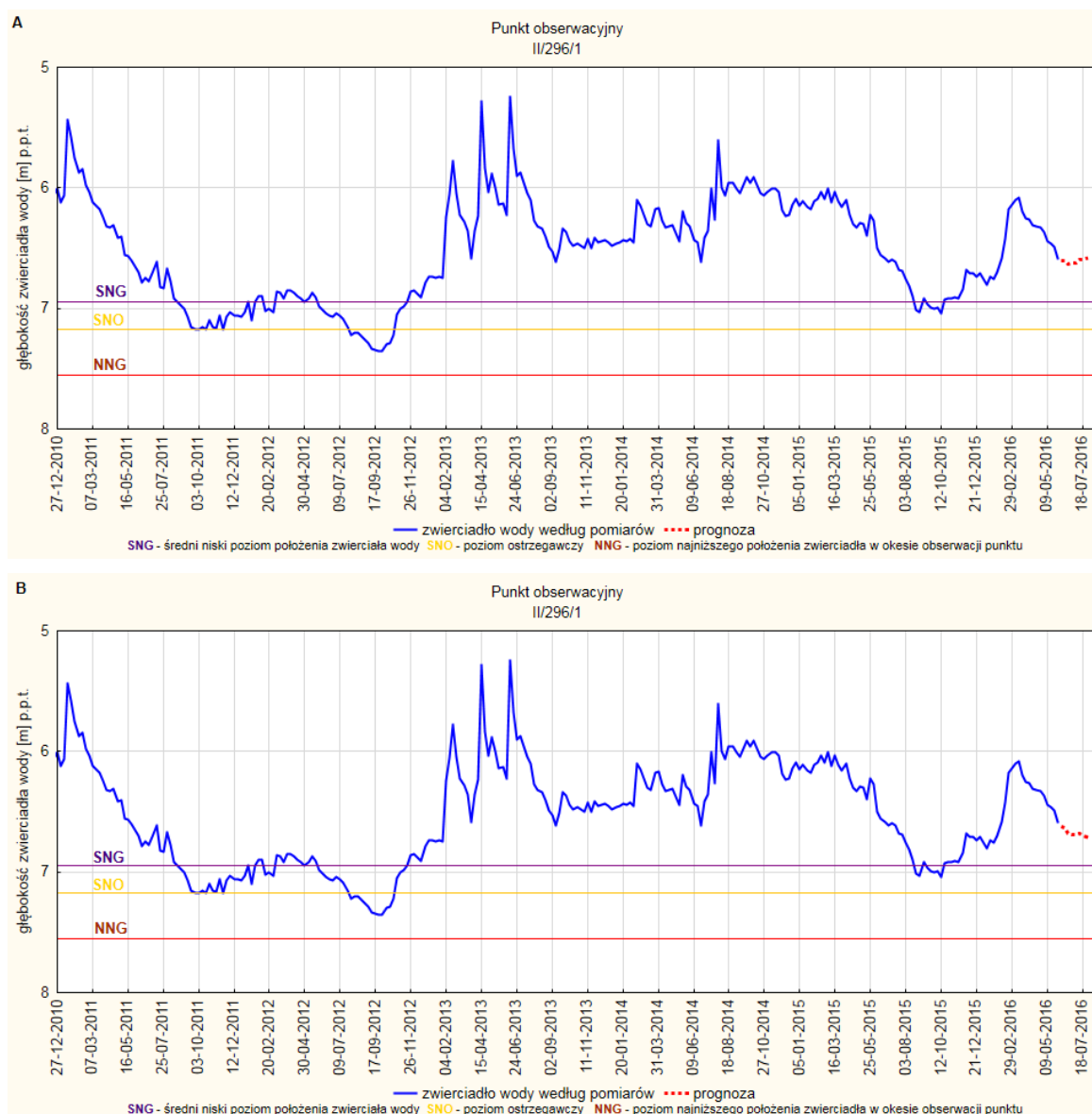
Rys. 32. Prognoza dotycząca stanu wód o zwierciadle swobodnym (gruntowych) na okres 01.07-31.07.2016 r. – stacja hydrogeologiczna nr II/296/1 w miejscowości Goleniowy (woj. śląskie). A - prognoza przy założeniu scenariusza A; B - prognoza przy założeniu scenariusza B
