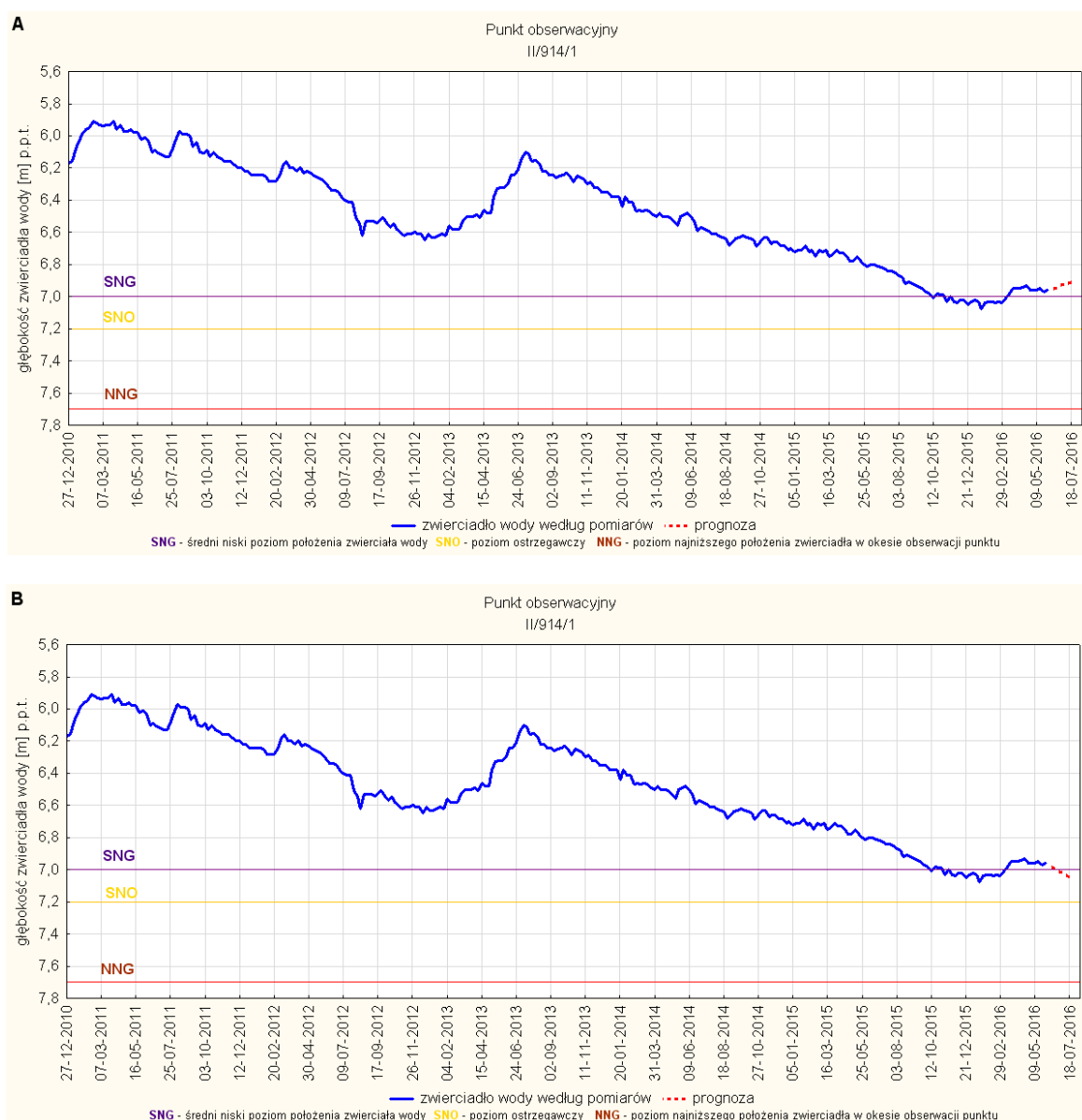
Rys. 16. Prognoza dotycząca stanu wód o zwierciadle swobodnym (gruntowych) na okres 01.07-31.07.2016r. – stacja hydrogeologiczna nr II/914/1 w miejscowości Bogdaszowice (woj. dolnośląskie). A - prognoza przy założeniu scenariusza A; B - prognoza przy założeniu scenariusza B
