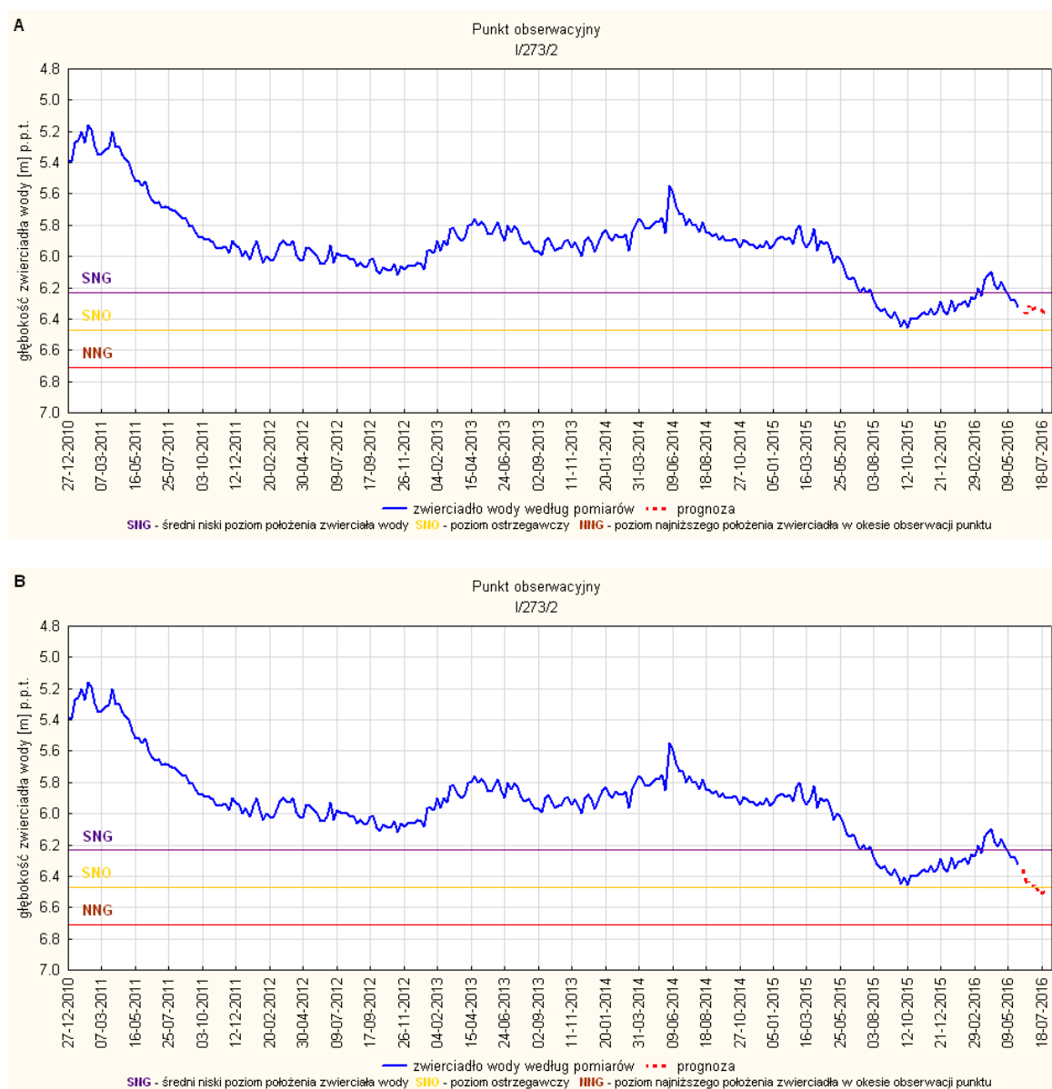
Rys. 9. Prognoza dotycząca stanu wód o zwierciadle swobodnym (gruntowych) na okres 01.07-31.07.2016r. – stacja hydrogeologiczna nr I/273/2 w miejscowości Sarbicko (woj. wielkopolskie). A - prognoza przy założeniu scenariusza A; B - prognoza przy założeniu scenariusza B
