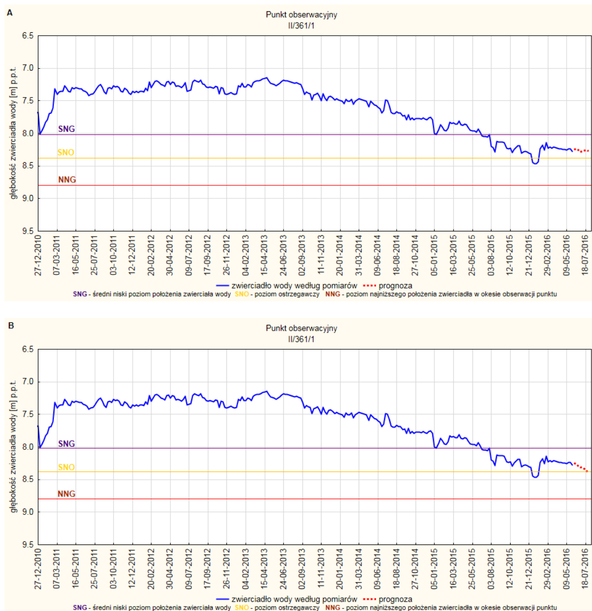
Rys. 3. Prognoza dotycząca stanu wód o zwierciadle swobodnym (gruntowych) na okres 01.07-31.07.2016r. – stacja hydrogeologiczna nr II/361/1 w Murzynie (woj. lubuskie). A - prognoza przy założeniu scenariusza A; B - prognoza przy założeniu scenariusza B
