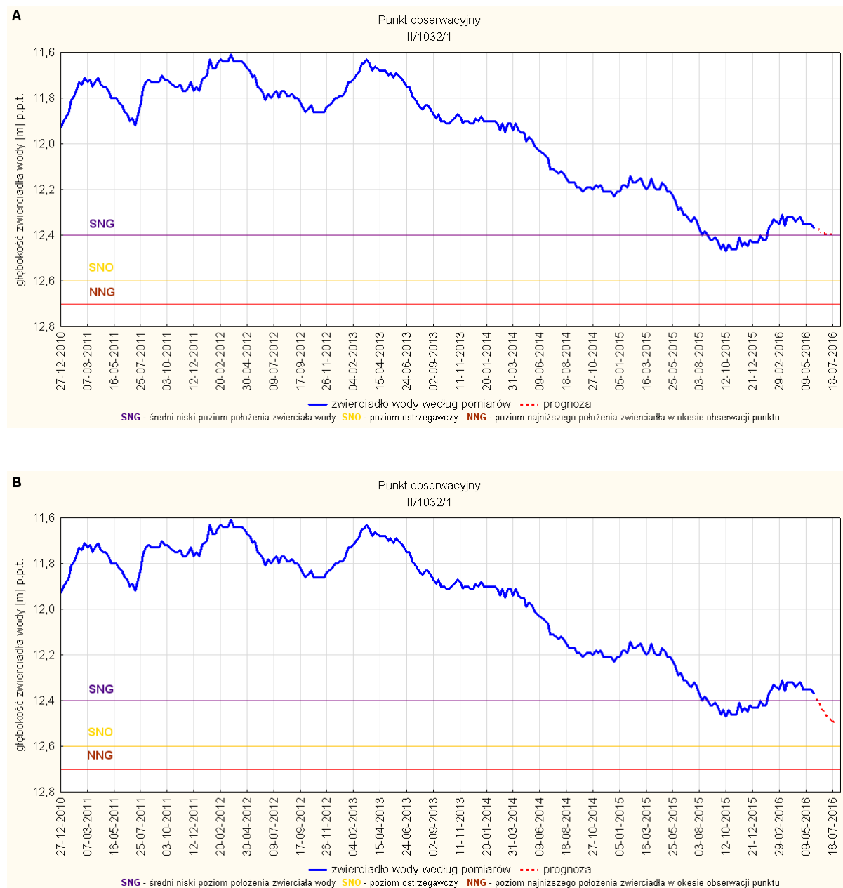
Rys. 2. Prognoza dotycząca stanu wód o zwierciadle swobodnym (gruntowych) na okres 01.07-31.07.2016r. – stacja hydrogeologiczna nr II/1032/1 w Gądnie (woj. zachodniopomorskie). A - prognoza przy założeniu scenariusza A; B - prognoza przy założeniu scenariusza B
