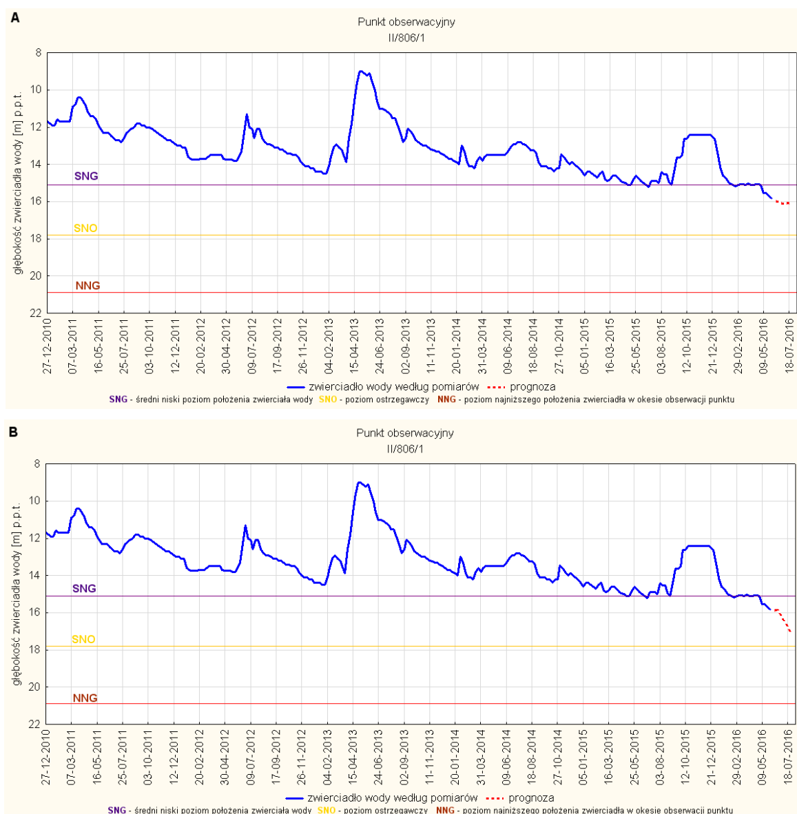
Rys. 21. Prognoza dotycząca stanu wód o zwierciadle swobodnym (gruntowych) na okres 01.07-31.07.2016r. – stacja hydrogeologiczna nr II/806/1 w Mokłuczce (woj. podkarpackie). A - prognoza przy założeniu scenariusza A; B - prognoza przy założeniu scenariusza B
