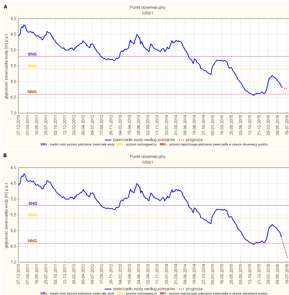
Rys. 14. Prognoza dotycząca stanu wód o zwierciadle swobodnym (gruntowych) na okres 01.07-31.07.2016r. – stacja hydrogeologiczna nr II/80/1 w Ciechanowie (woj. mazowieckie). A - prognoza przy założeniu scenariusza A; B - prognoza przy założeniu scenariusza B
