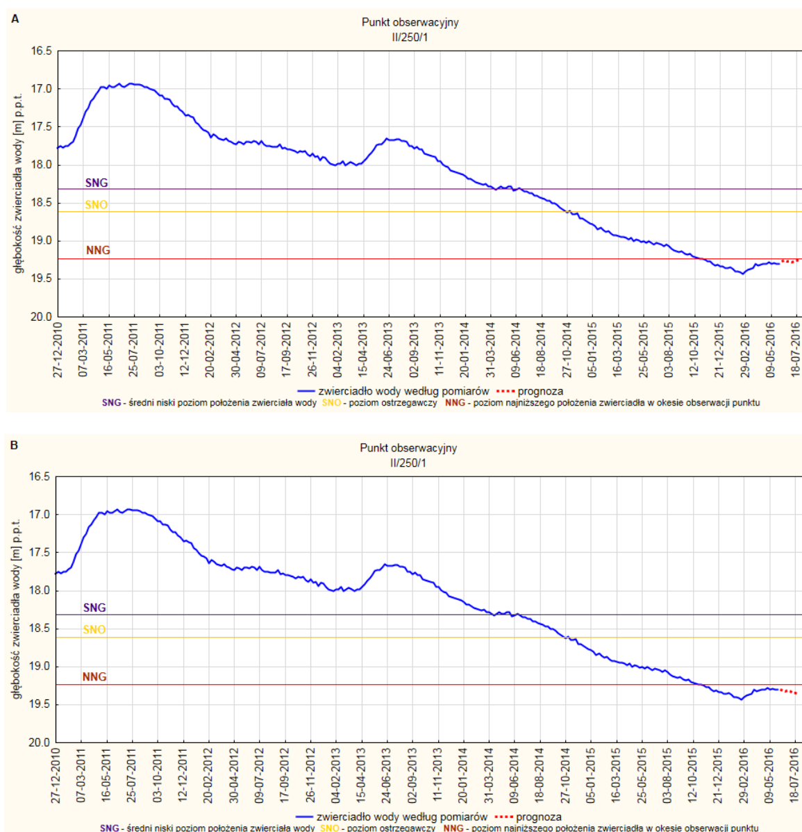
Rys. 23. Prognoza dotycząca stanu wód o zwierciadle swobodnym (gruntowych) na okres 01.07-31.07.2016r. – stacja hydrogeologiczna nr II/250/1 w Kobałtach (woj. warmińsko-mazurskie). A - prognoza przy założeniu scenariusza A; B - prognoza przy założeniu scenariusza B
