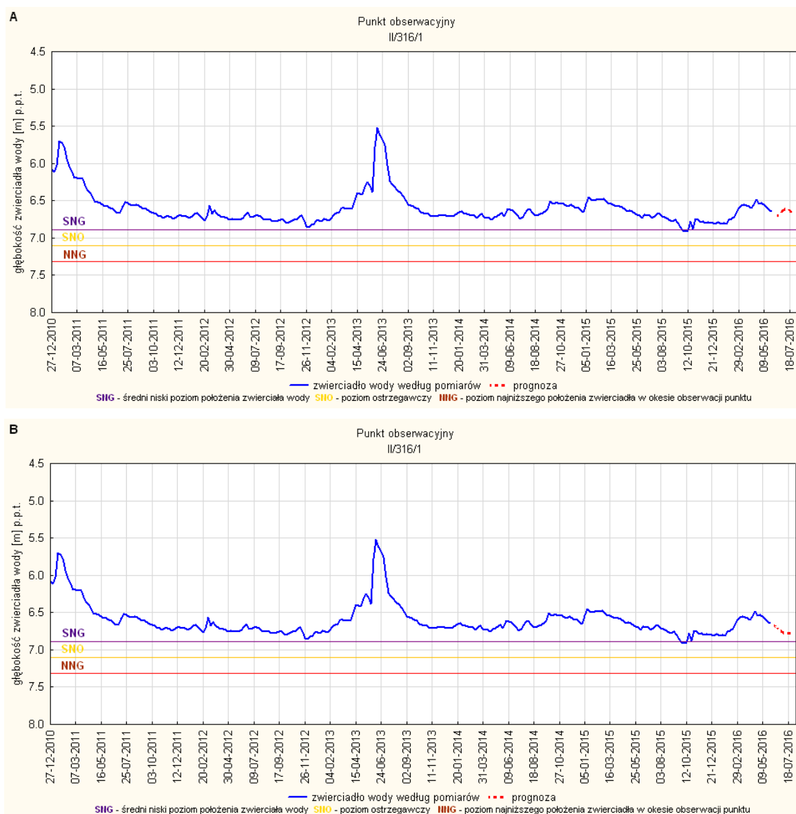
Rys. 25. Prognoza dotycząca stanu wód o zwierciadle swobodnym (gruntowych) na okres 01.07-31.07.2016r. – stacja hydrogeologiczna nr II/316/1 w Masłowicach (woj. łódzkie). A - prognoza przy założeniu scenariusza A; B - prognoza przy założeniu scenariusza B
