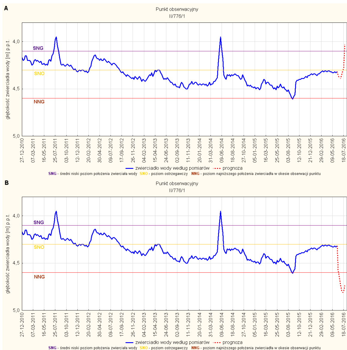
Rys. 27. Prognoza dotycząca stanu wód o zwierciadle swobodnym (gruntowych) na okres 01.07-31.07.2016r. – stacja hydrogeologiczna nr II/776/1 w Nowym Sączu (woj. małopolskie). A - prognoza przy założeniu scenariusza A; B - prognoza przy założeniu scenariusza B
