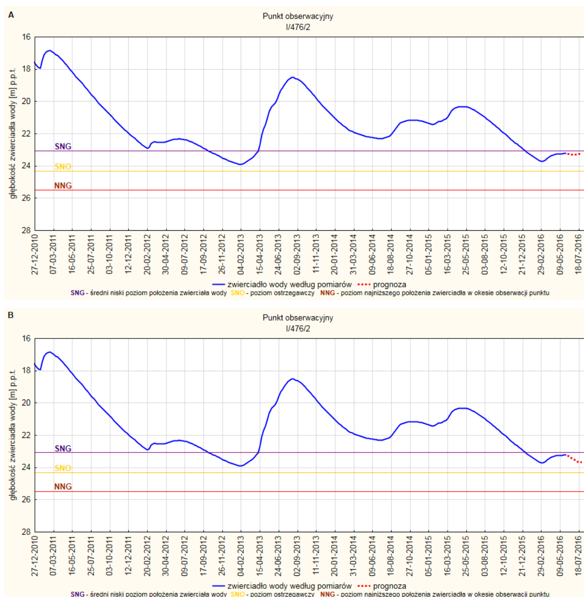
Rys. 30. Prognoza dotycząca stanu wód o zwierciadle swobodnym (gruntowych) na okres 01.07-31.07.2016 r. – stacja hydrogeologiczna nr I/476/2 w miejscowości Morusy (woj. śląskie). A - prognoza przy założeniu scenariusza A; B - prognoza przy założeniu scenariusza B
