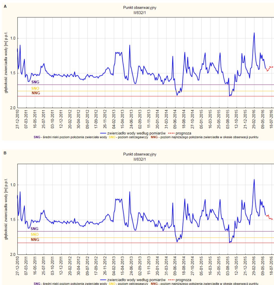
Rys. 28. Prognoza dotycząca stanu wód o zwierciadle swobodnym (gruntowych) na okres 01.07-31.07.2016r. – stacja hydrogeologiczna nr II/832/1 w Lubasz (woj. małopolskie). A - prognoza przy założeniu scenariusza A; B - prognoza przy założeniu scenariusza B
