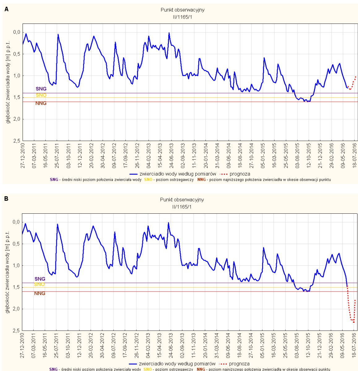
Rys. 17. Prognoza dotycząca stanu wód o zwierciadle swobodnym (gruntowych) na okres 01.07-31.07.2016r. – stacja hydrogeologiczna nr II/1165/1 w miejscowości Zgorzelec (woj. dolnośląskie). A - prognoza przy założeniu scenariusza A; B - prognoza przy założeniu scenariusza B
