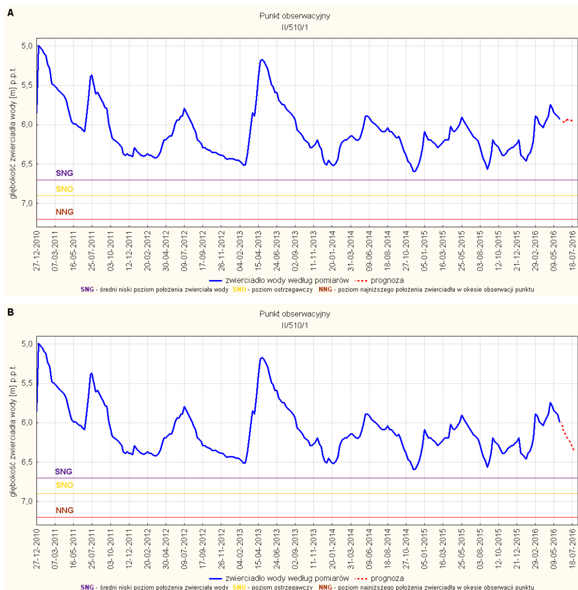
Rys. 29. Prognoza dotycząca stanu wód o zwierciadle swobodnym (gruntowych) na okres 01.07-31.07.2016r. – stacja hydrogeologiczna nr II/510/1 w miejscowości Siemień (woj. lubelskie). A - prognoza przy założeniu scenariusza A; B - prognoza przy założeniu scenariusza B
