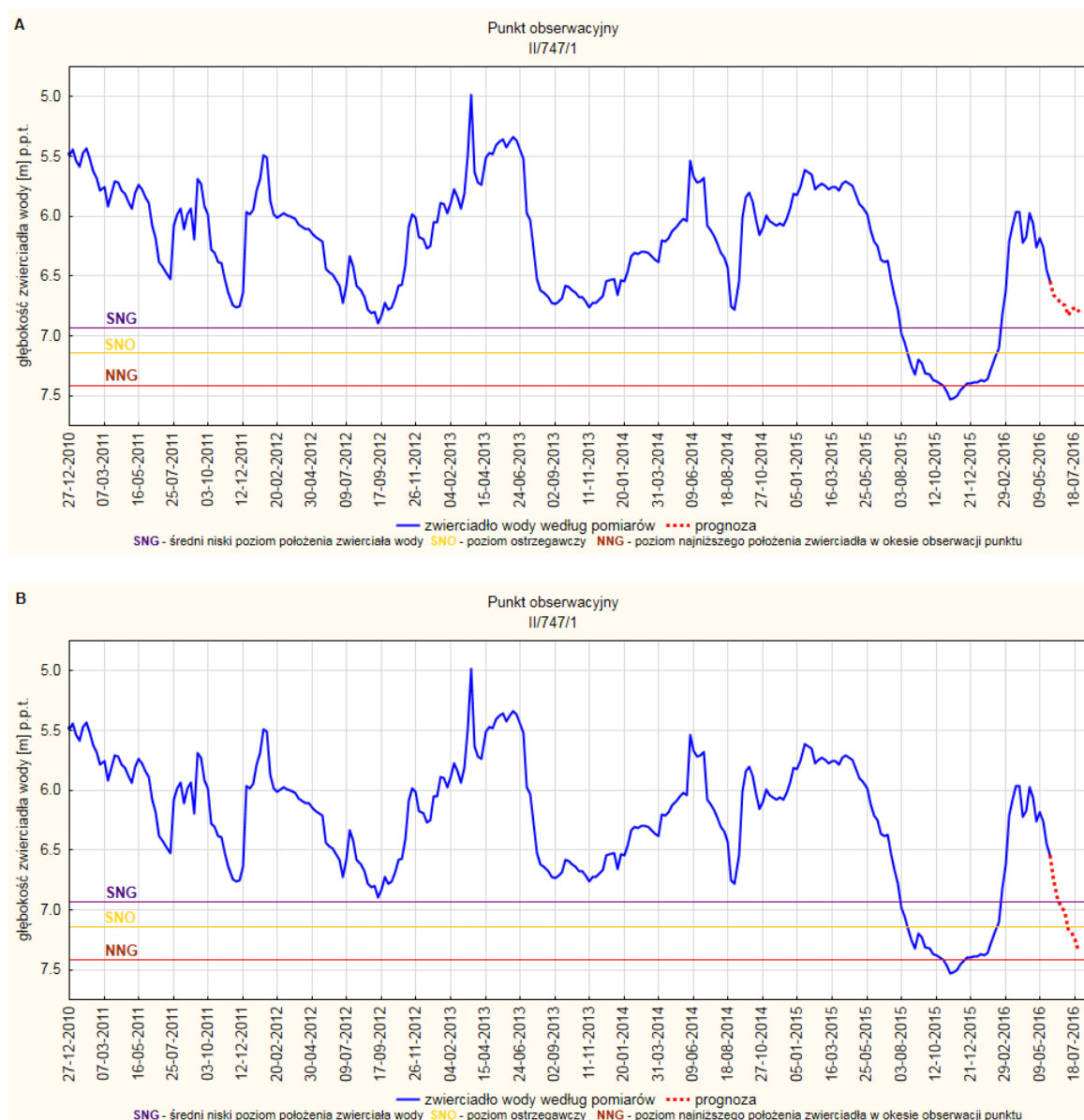
Rys. 15. Prognoza dotycząca stanu wód o zwierciadle swobodnym (gruntowych) na okres od 01.07-31.07.2016r. – stacja hydrogeologiczna nr II/747/1 w miejscowości Stary Wielisław (woj. dolnośląskie). A - prognoza przy założeniu scenariusza A; B - prognoza przy założeniu scenariusza
