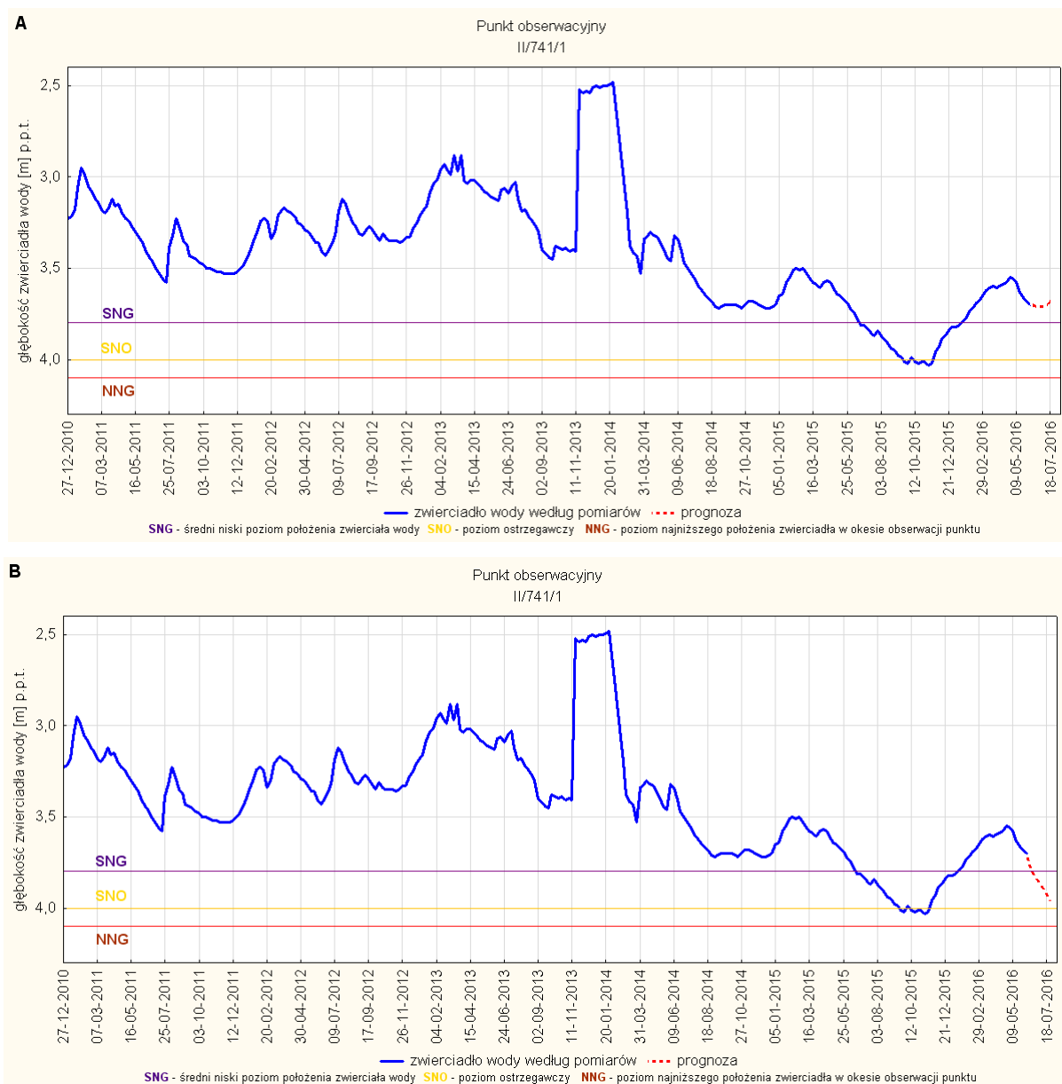
Rys. 6. Prognoza dotycząca stanu wód o zwierciadle swobodnym (gruntowych) na okres 01.07-31.07.2016r. – stacja hydrogeologiczna nr II/741/1 w Kiełpinie (woj. lubuskie). A - prognoza przy założeniu scenariusza A; B - prognoza przy założeniu scenariusza B
