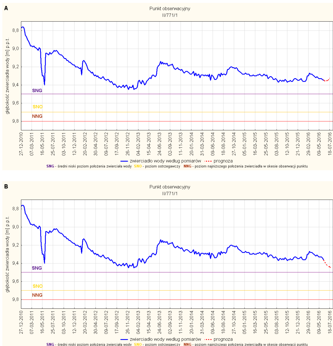
Rys. 26. Prognoza dotycząca stanu wód o zwierciadle swobodnym (gruntowych) na okres 01.07-31.07.2016r. – stacja hydrogeologiczna nr II/771/1 w Krakowie (woj. małopolskie). A - prognoza przy założeniu scenariusza A; B - prognoza przy założeniu scenariusza B
