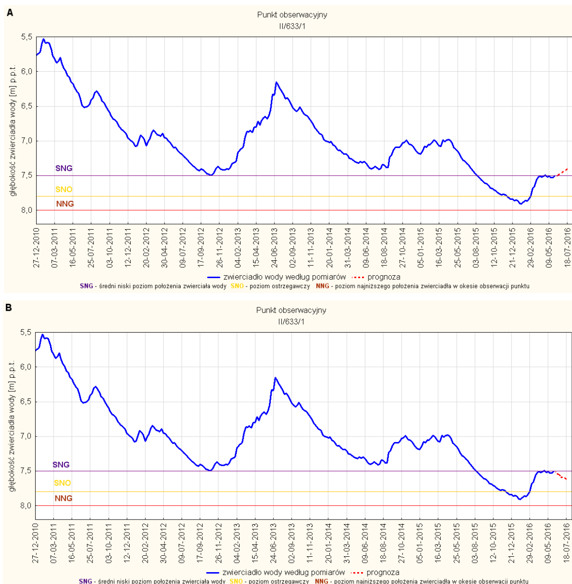
Rys. 22. Prognoza dotycząca stanu wód o zwierciadle swobodnym (gruntowych) na okres 01.07-31.07.2016r. – stacja hydrogeologiczna nr II/633/1 w miejscowości Łącznik (woj. opolskie). A - prognoza przy założeniu scenariusza A; B - prognoza przy założeniu scenariusza B
