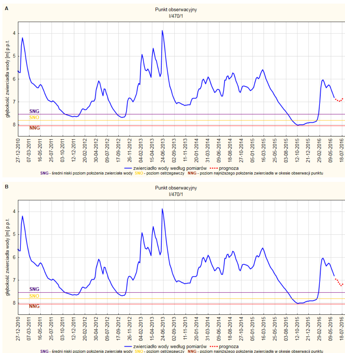
Rys. 31. Prognoza dotycząca stanu wód o zwierciadle swobodnym (gruntowych) na okres 01.07-31.07.2016 r. – stacja hydrogeologiczna nr I/470/1 w miejscowości Podlesie (woj. śląskie). A - prognoza przy założeniu scenariusza A; B - prognoza przy założeniu scenariusza
