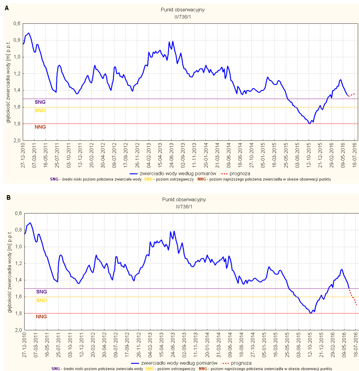
Rys. 5. Prognoza dotycząca stanu wód o zwierciadle swobodnym (gruntowych) na okres 01.07-31.07.2016r. – stacja hydrogeologiczna nr II/736/1 w miejscowości Nowe Żabno (woj. lubuskie). A - prognoza przy założeniu scenariusza A; B - prognoza przy założeniu scenariusza B
