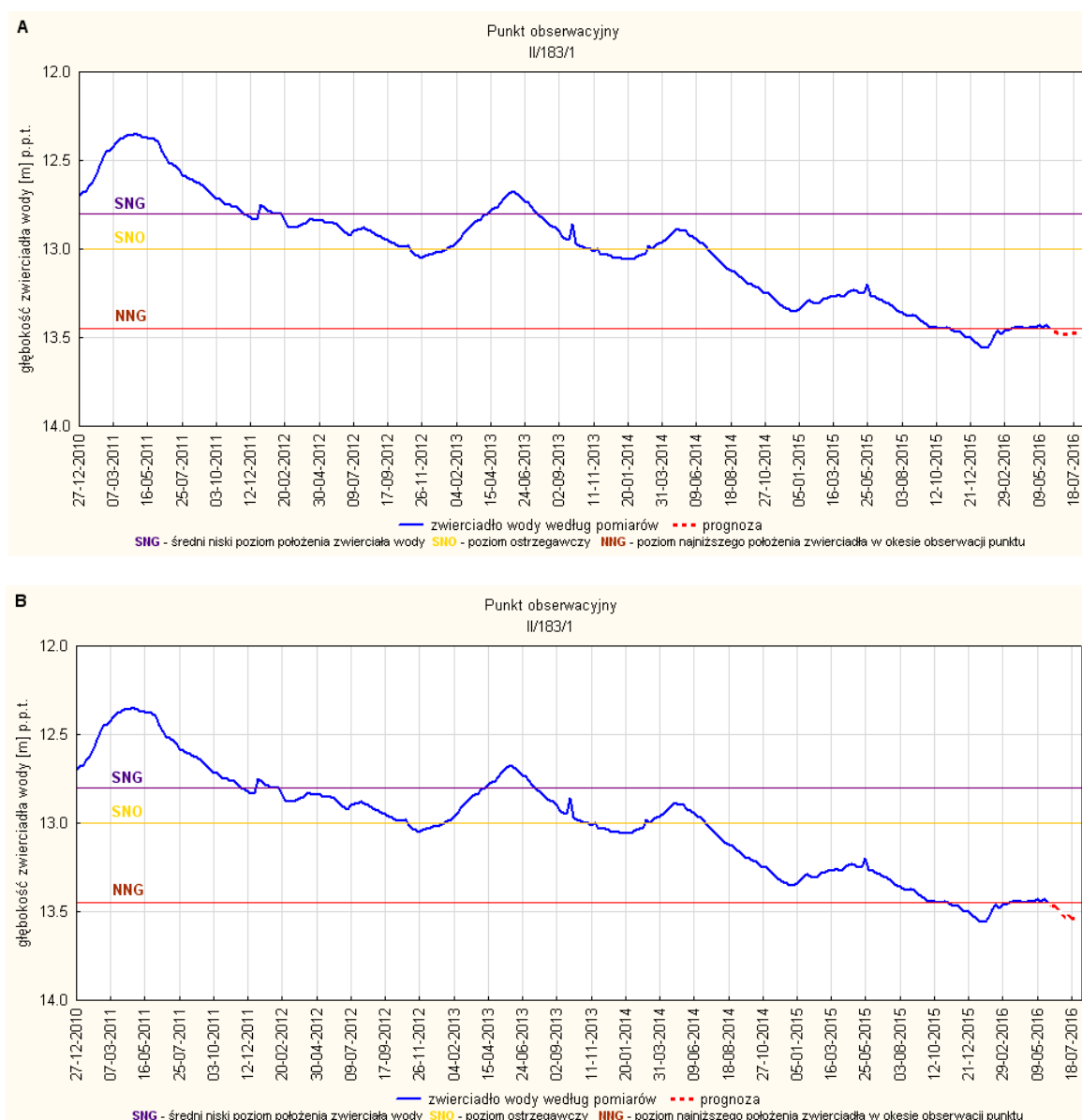
Rys. 11. Prognoza dotycząca stanu wód o zwierciadle swobodnym (gruntowych) na okres 01.07-31.07.2016r. – stacja hydrogeologiczna II/183/1 Wierzychy (woj. kujawsko-pomorskie). A - prognoza przy założeniu scenariusza A; B - prognoza przy założeniu scenariusza B
