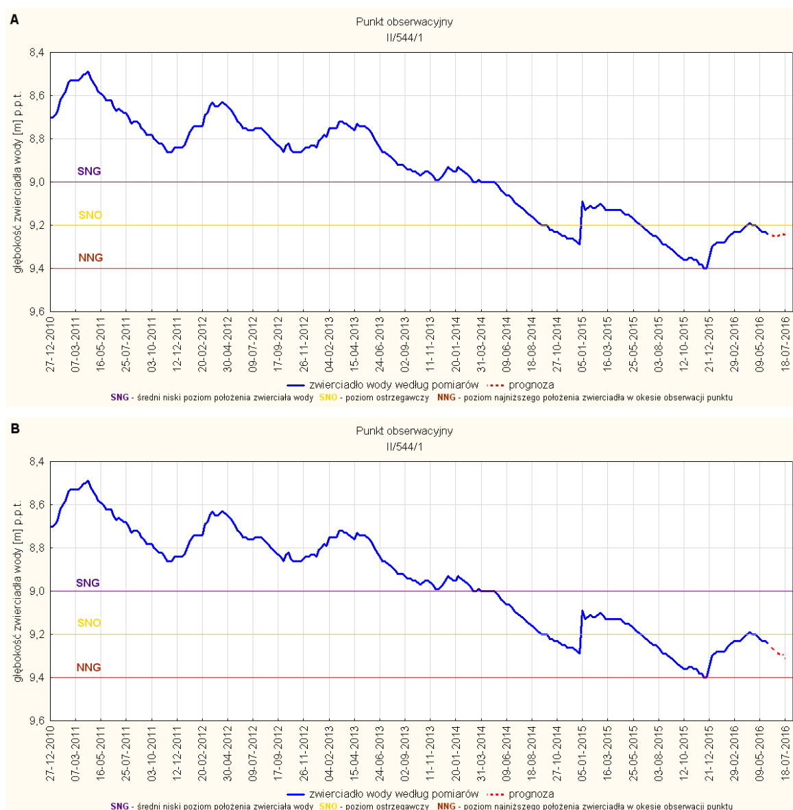
Rys. 24. Prognoza dotycząca stanu wód o zwierciadle swobodnym (gruntowych) na okres 01.07-31.07.2016r. – stacja hydrogeologiczna nr II/544/1 w Łysomiczkach (woj. pomorskie). A - prognoza przy założeniu scenariusza A; B - prognoza przy założeniu scenariusza B
