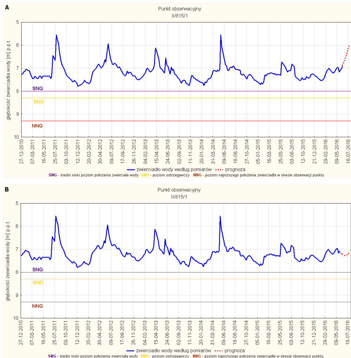
Rys. 20. Prognoza dotycząca stanu wód o zwierciadle swobodnym (gruntowych) na okres 01.07-31.07.2016r. – stacja hydrogeologiczna nr II/815/1 w miejscowości Lesko (woj. podkarpackie). A - prognoza przy założeniu scenariusza A; B - prognoza przy założeniu scenariusza B
