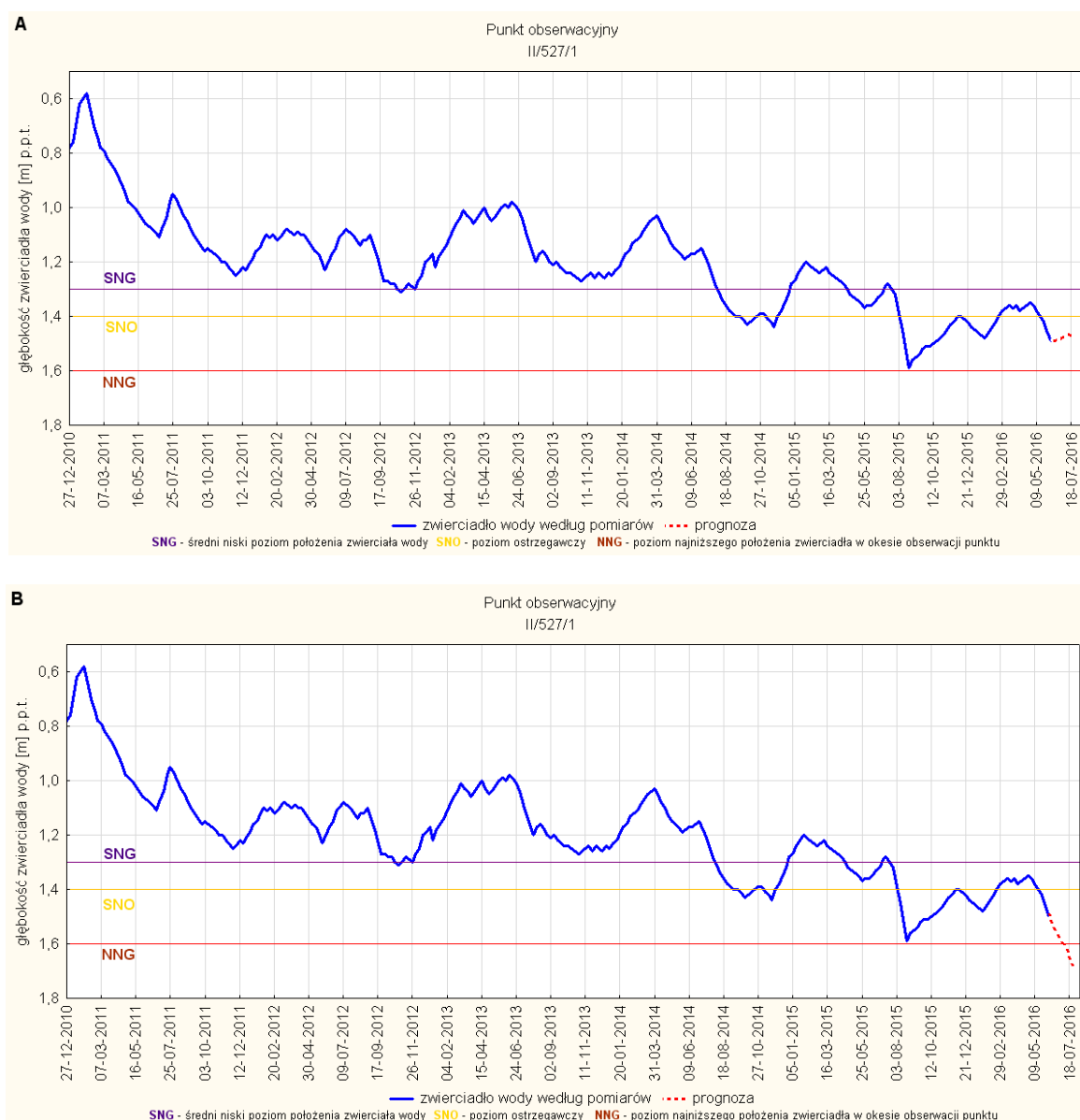
Rys. 12. Prognoza dotycząca stanu wód o zwierciadle swobodnym (gruntowych) na okres 01.07-31.07.2016r. – stacja hydrogeologiczna II/527/1 Szubin (woj. kujawsko-pomorskie). A - prognoza przy założeniu scenariusza A; B - prognoza przy założeniu scenariusza B
