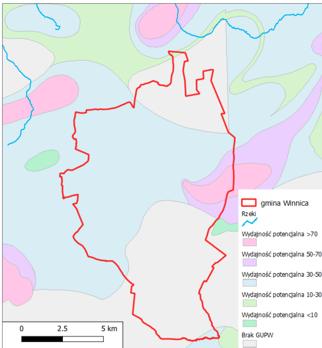
Rysunek 23 Wydajność potencjalna studni wierconej na terenie gminy Winnica
