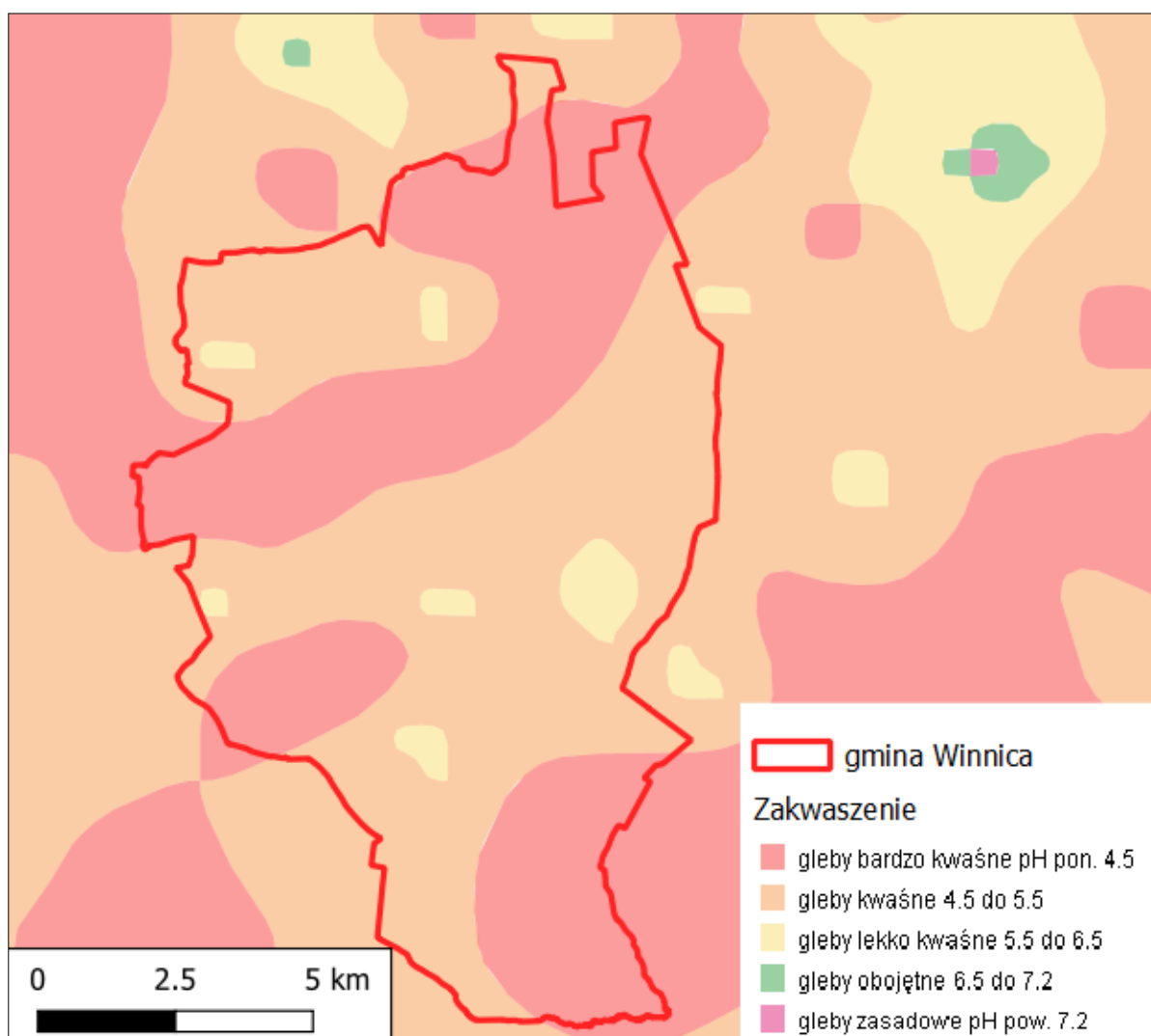
Rysunek 32. Położenie Gminy Winnica na tle mapy zakwaszenia gleb
